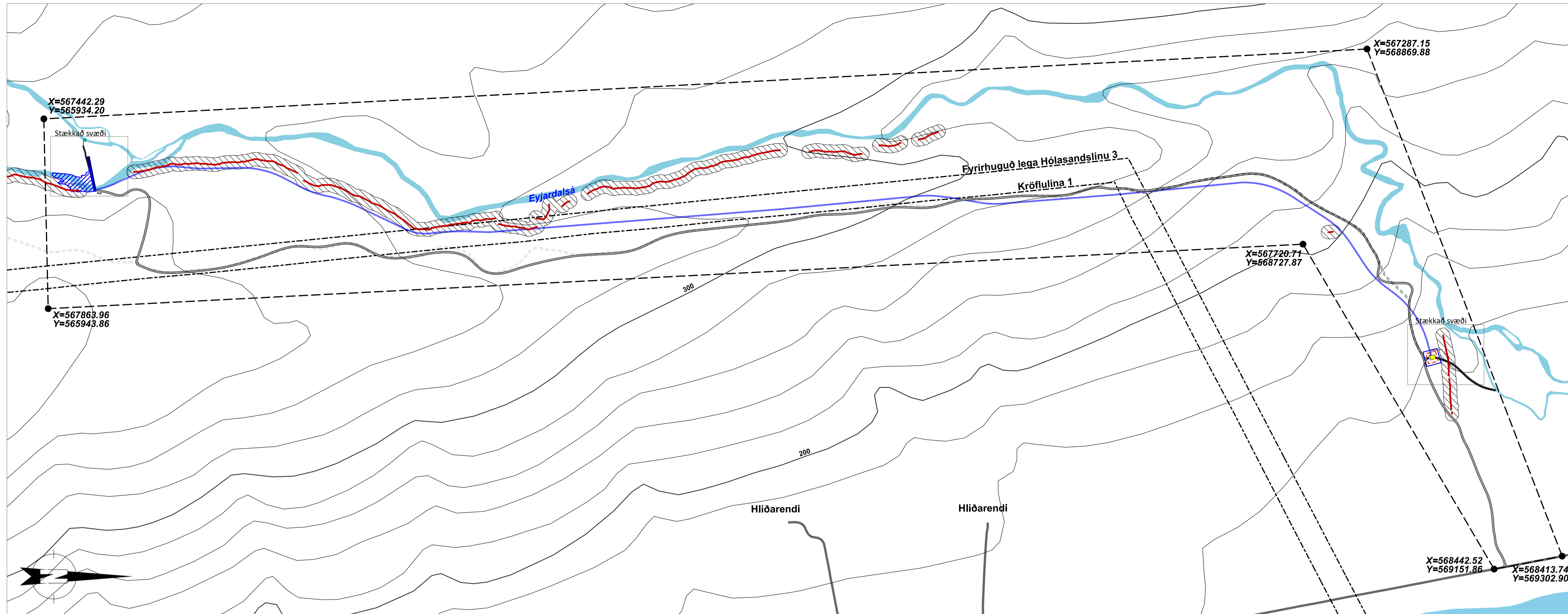
Deiliskipulag, mvk. 1:5.000
