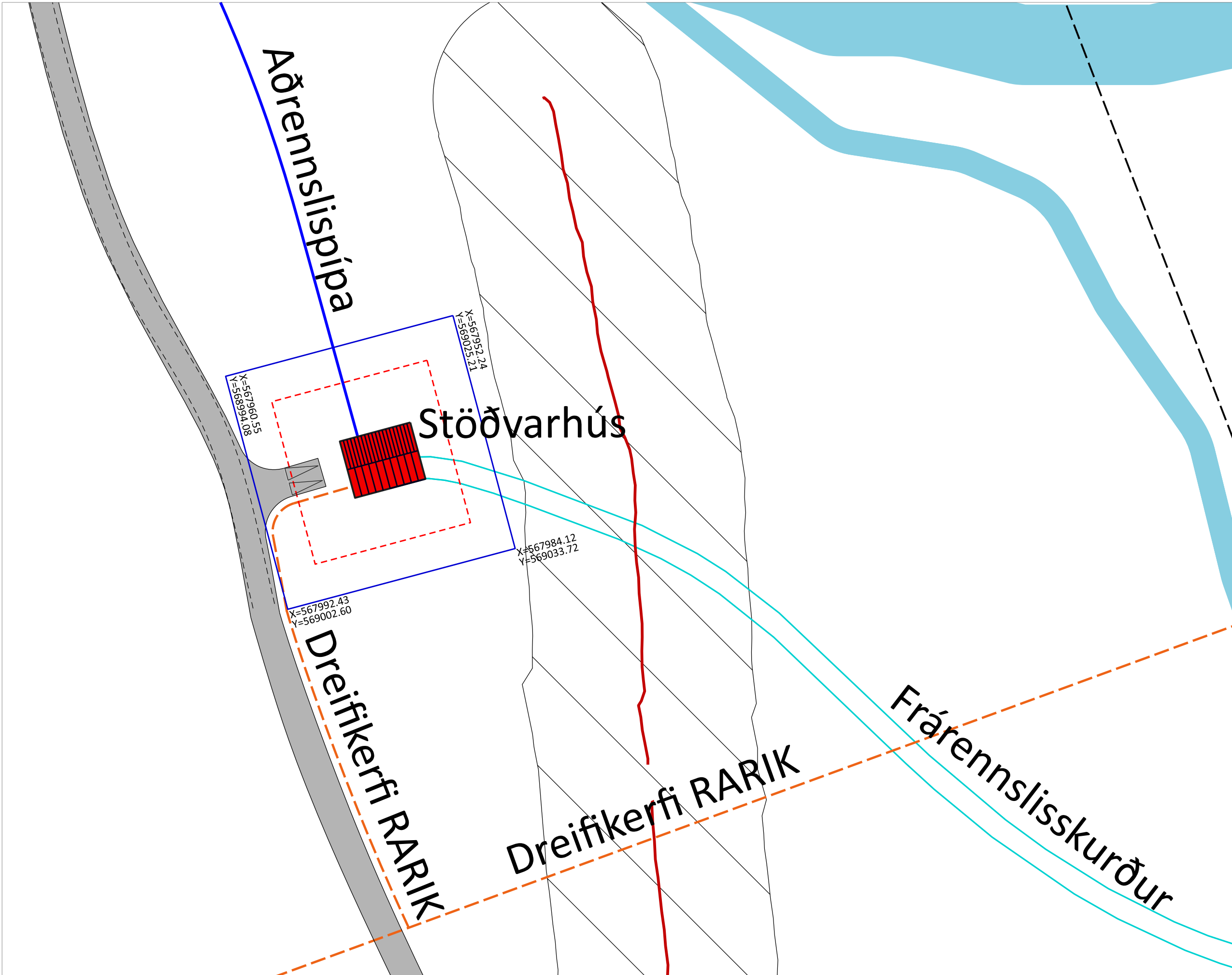
Stöðvarhús, mvk. 1:500
