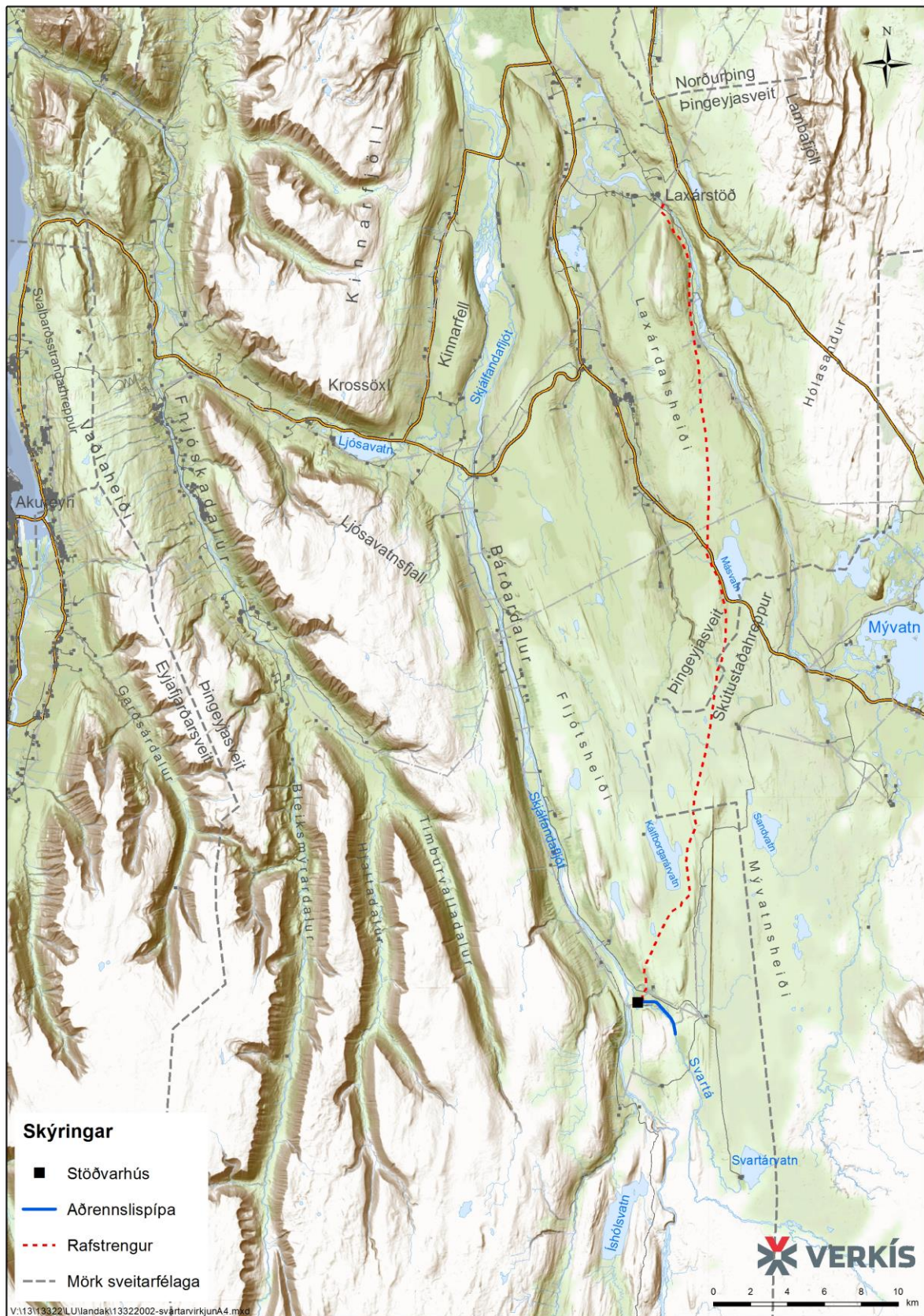
Mynd 1.1 Fyrirhuguð staðsetning virkjunar og stöðvarhúss auk jarðstrengs sýnd á skýringarupprætti
